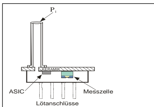
Abbildung 6: Absolutdrucksensor am Beispiel AMS 5812 [3]
